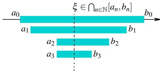
FIGURE I.8 – Propriété des intervalles emboîtés
