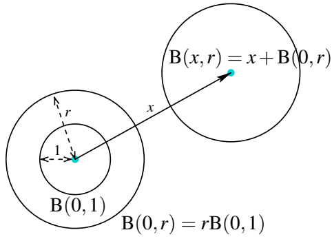
FIGURE II.5 – Translation et dilatation de la boule unité
