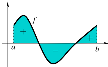
FIGURE VI.1 – Intégrale de f
