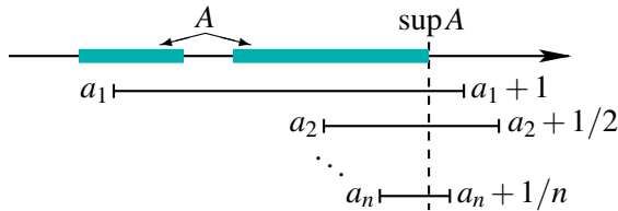
FIGURE I.7 – Suite croissante (a_n) convergeant vers le supremum
