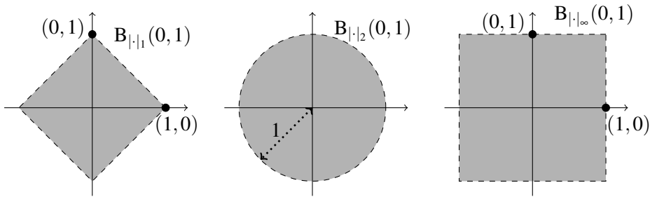
FIGURE II.6 – Boules unité ouvertes
