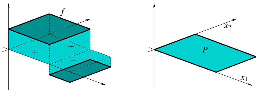
FIGURE VI.8 – Intégrale d'une fonction à deux variables
