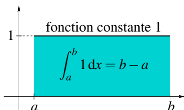
FIGURE VI.7 – Longueur d'un intervalle
