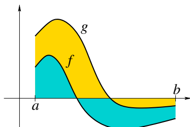
FIGURE VI.6 – Croissance de l'intégrale
