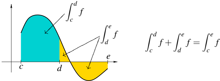
FIGURE VI.5 – Additivité de l'intégrale
