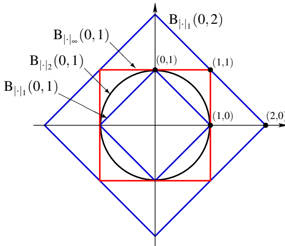
FIGURE II.7 – Inclusion des boules unités
